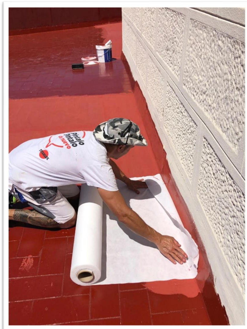
Colocación del velo sobre la primera mano de Imperpol
